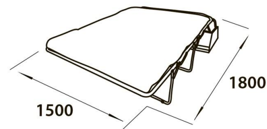
Спальное место диванной секции Механизм „Сюзи“
